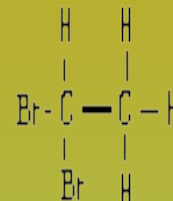
1,1-дибромэтан
