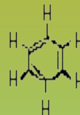
бензол
