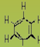
бензол
