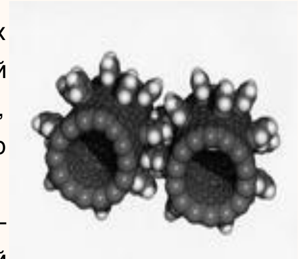
Молекула воска
