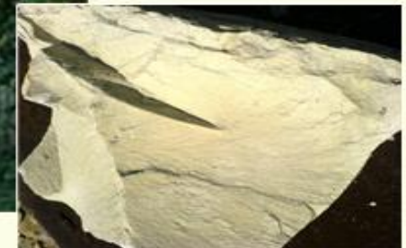
известняк ( \text{CaCO}_3 )
