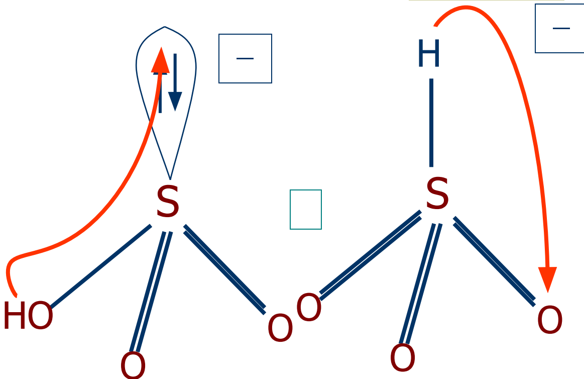
Гидросульфит-ион: таутомерия
