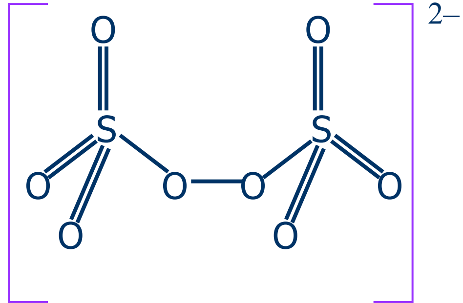
Пероксодисульфат-ион \text{S}_2\text{O}_6(\text{O}_2)^{2-}
