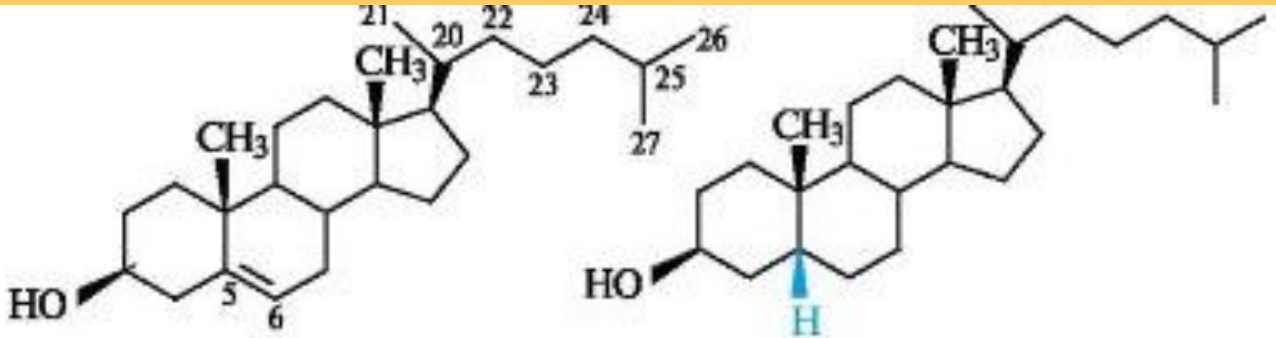
холестерин
