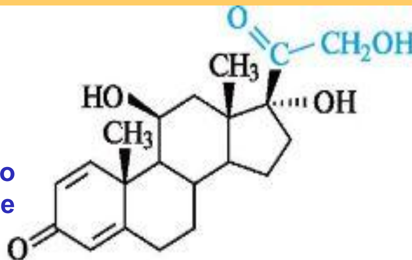
преднизолон
