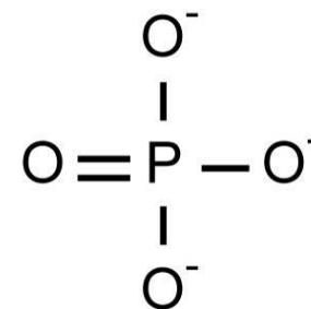
Фосфат-анион
