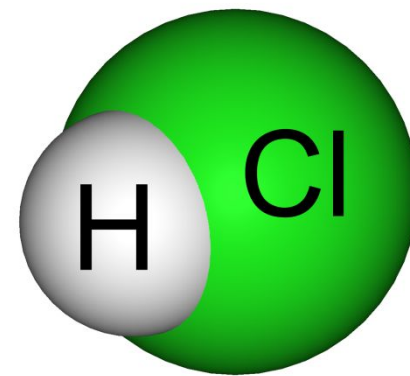
Хлоридная кислота
