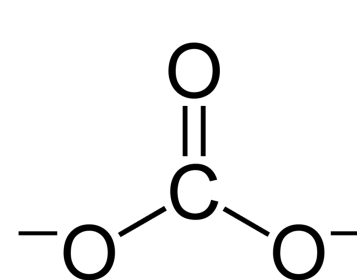
Карбонат-анион
