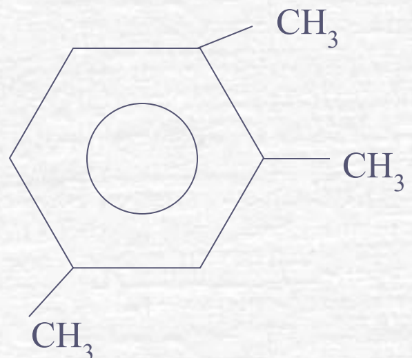
1,2,4-триметилбензол
