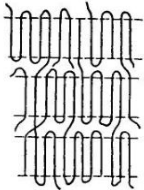
Схема соединения ламелей проходными молекулами и аморфные области между ламелями
