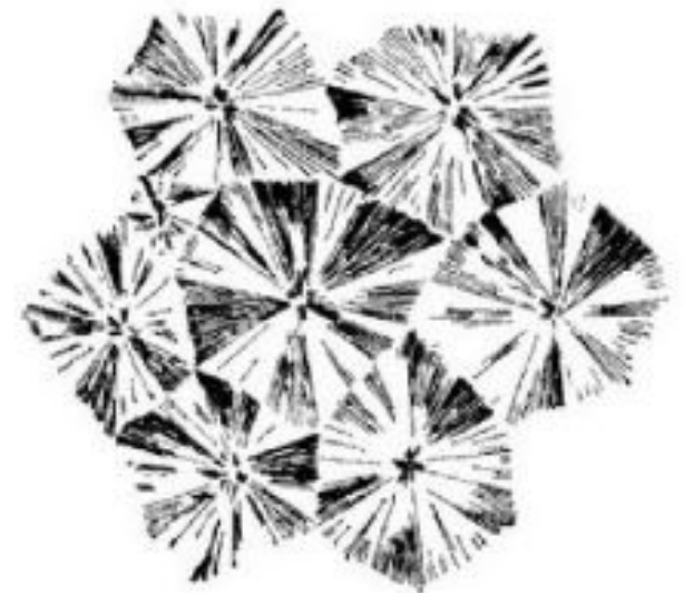
Фрагмент сферолитной структуры кристаллического термопласта (полипропилена)
