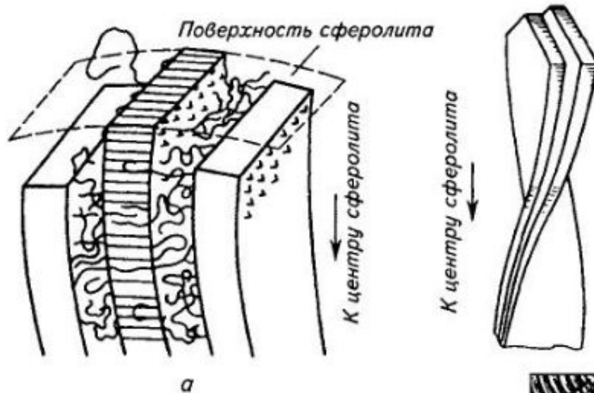
Рис. 10.4. Схема укладки макромолекул в сферолите. Располож альном ( a ) и кольцевом ( б ) сферолитах
