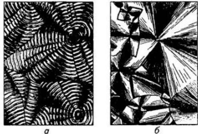
Рис. 10.5. Различные типы сферолитов:
