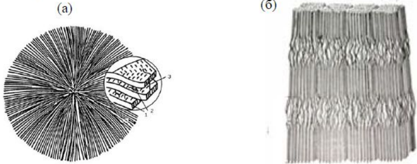
Рис. 3.20. Модель сферолита: 1 – ламель, 2 – межламелярная прослойка, 3 – проходная цепь (а); микрофибриллярная модель строения ориентированного полимера (б).
