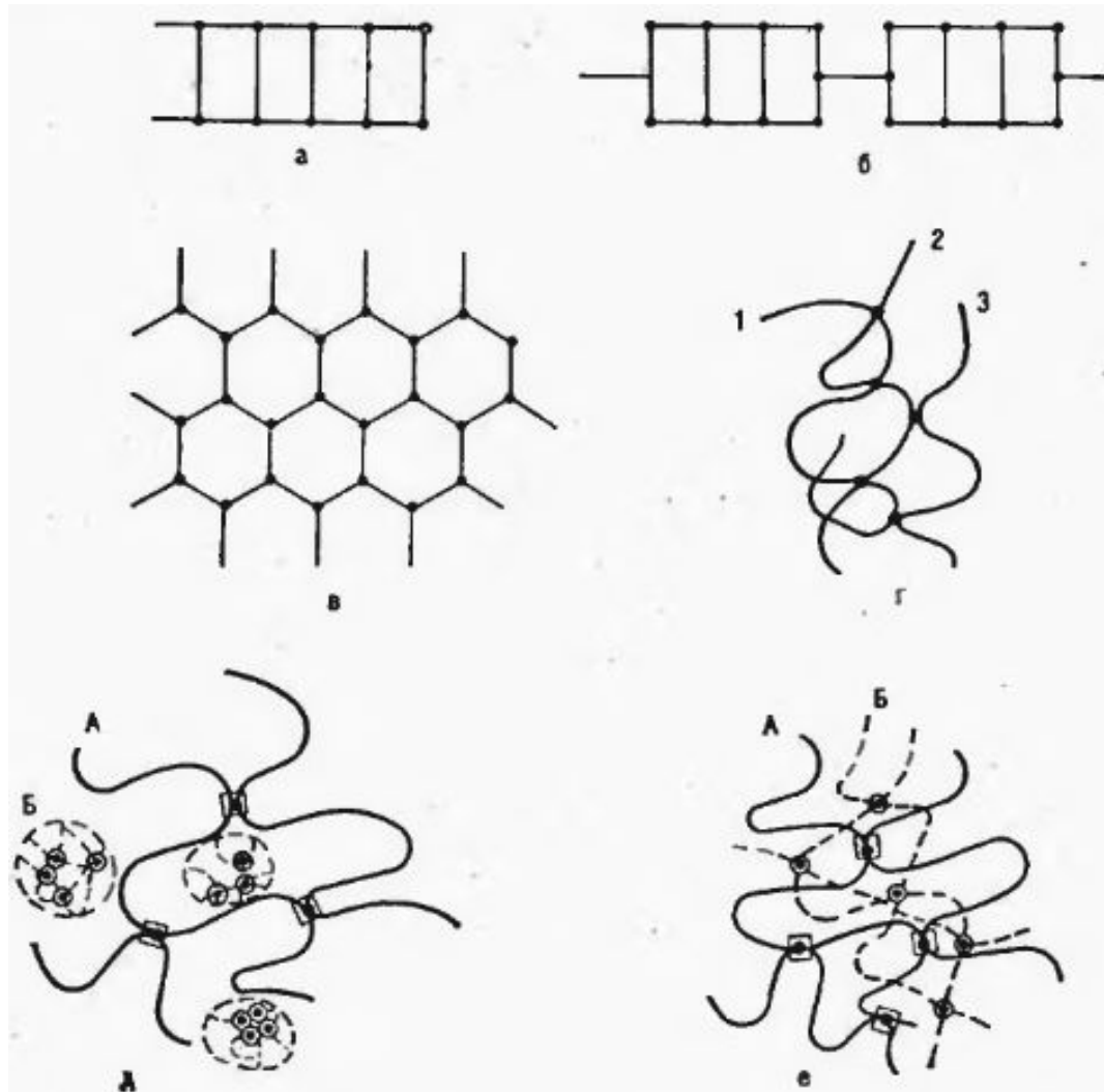
Рис.1.4. Схематическое изображение сетчатых полимеров: а – лестничные; б – полулестничные; в – плоскосетчатые; г – пространственно-сетчатые из одного полимера (1, 2, 3 – макромолекулы, темные точки – узлы); д, е – пространственно-сетчатые из полимера А (сплошные линии) и полимера Б (пунктир)
