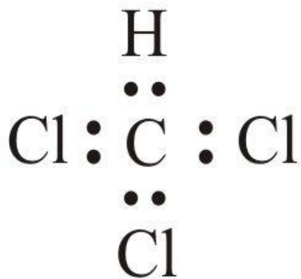
трихлорметан
