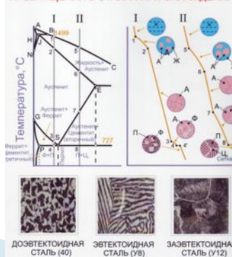
ПРЕВРАЩЕНИЯ В СТАЛЯХ ПРИ ОХЛАЖДЕНИИ
