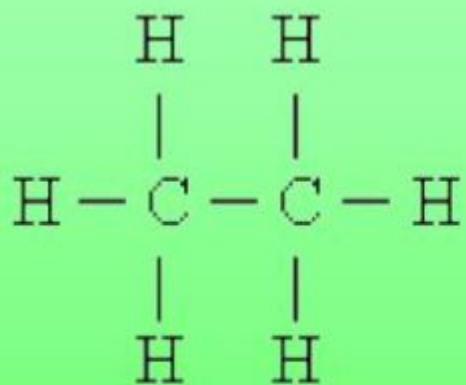
этан
