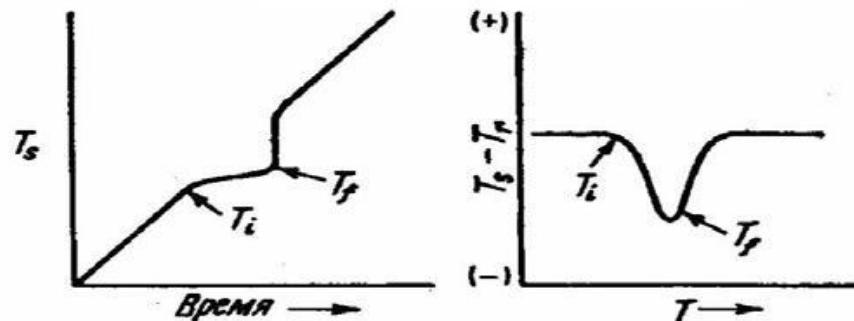
Эндотермическое превращение
