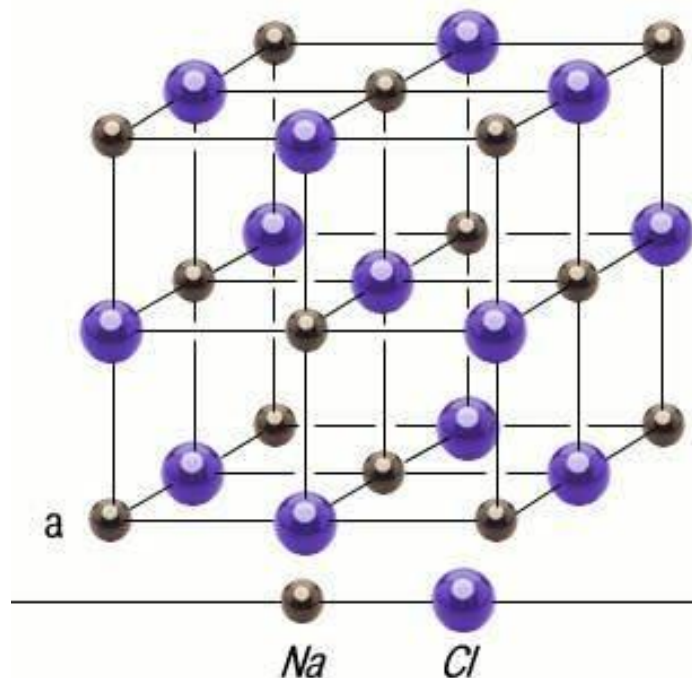
Кристалл поваренной соли NaCl
