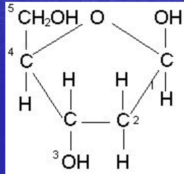
Дезоксирибоза
