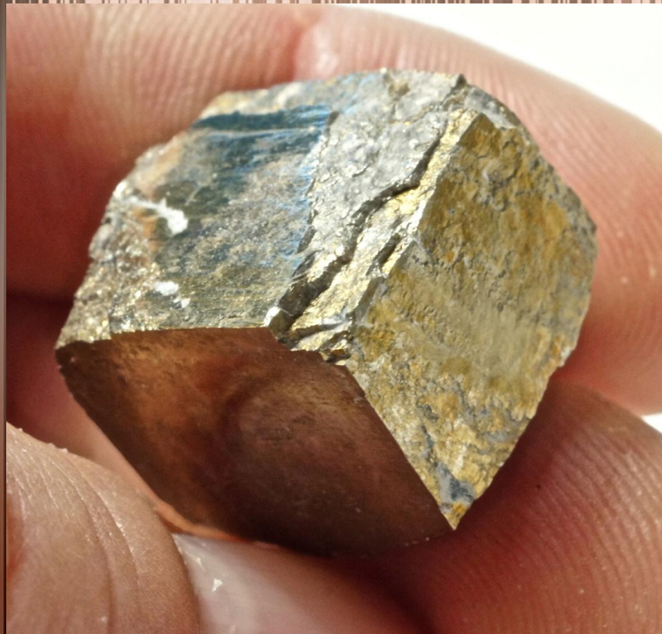
Самородная медь
