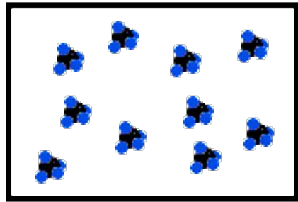
CH4 метан 16 г/моль
