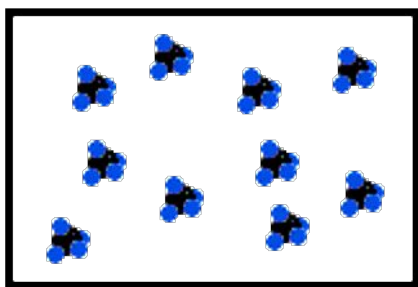
CH4 метан 16 г/моль
