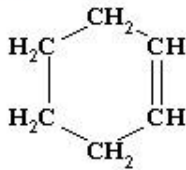
Циклогексен
