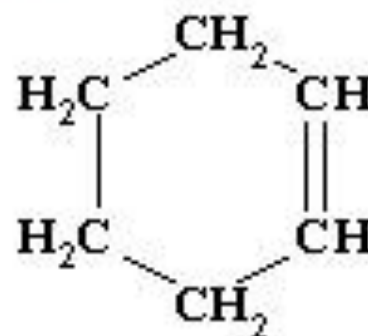
Циклогексен
