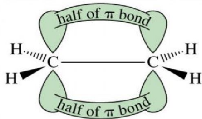
\pi -связь
