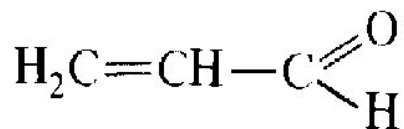
акролеин
