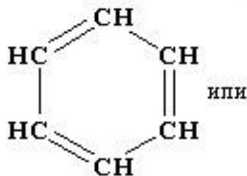
Бензол
