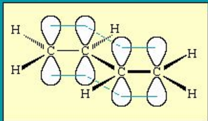
\text{CH}_2 = \text{CH} - \text{CH} = \text{CH}_2 бутадиен-1,3
