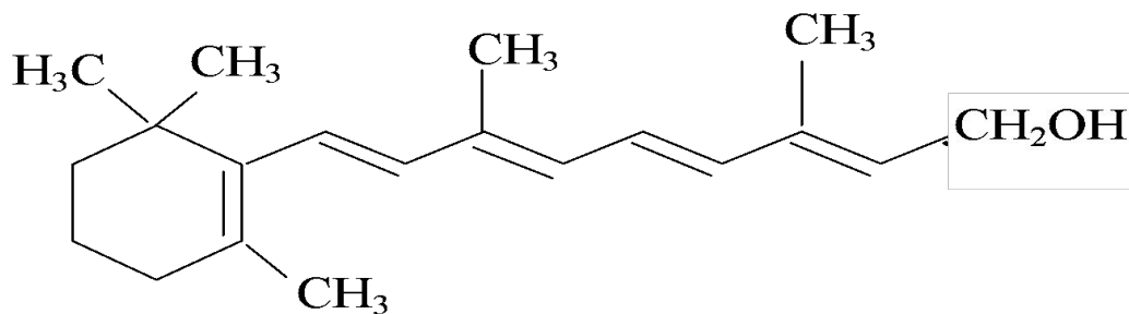
Ретинол (витаминА)
