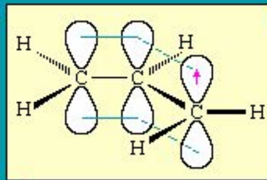
\text{CH}_2=\text{CH}-\dot{\text{C}}\text{H}_2 аллил-радикал
