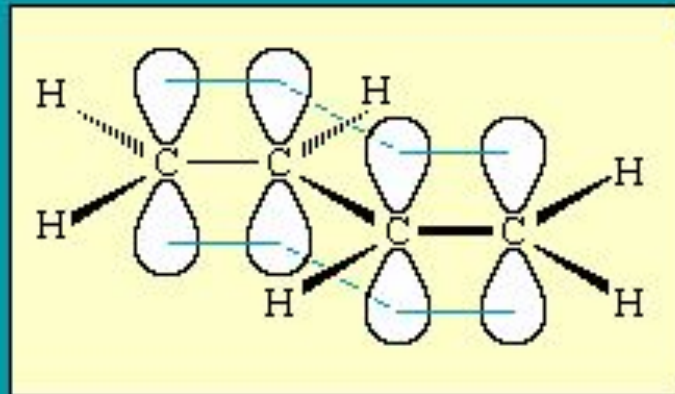
\text{CH}_2=\text{CH}-\text{CH}=\text{CH}_2 бутадиен-1,3
