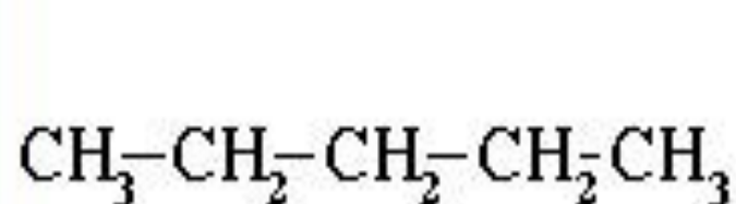
н-Пентан
