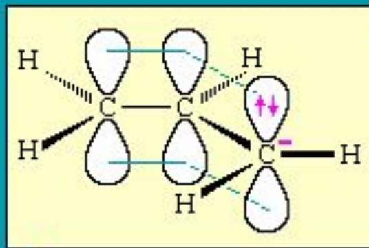
\text{CH}_2=\text{CH}-\overset{-}{\text{C}}\text{H}_2 аллил-анион
