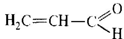
акролеин
