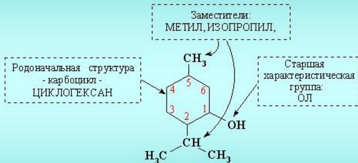
2-Изопропил-5-метилциклогексанол-1
