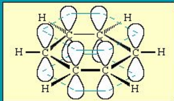
\text{C}_6\text{H}_6 бензол
