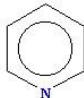
Пиридин
