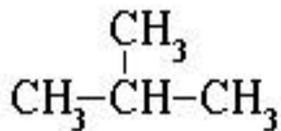
Изобутан
