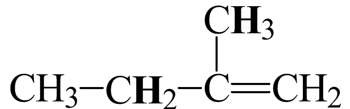
2-метилбутен-1
