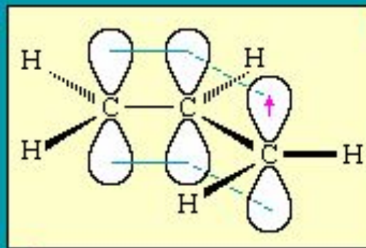
\text{CH}_2=\text{CH}-\dot{\text{C}}\text{H}_2 аллил-радикал
