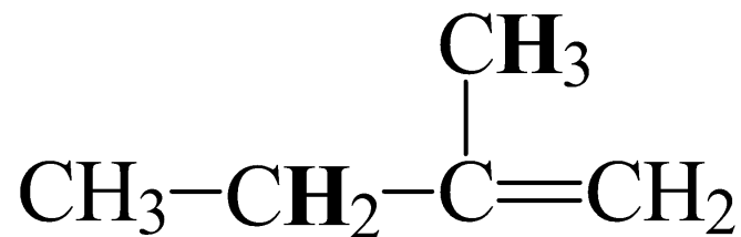
2-метилбутен-1
