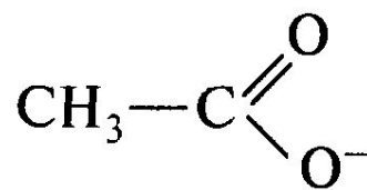
ацетат-ион
