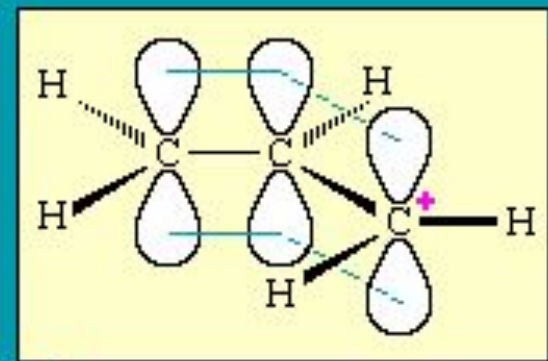
\text{CH}_2=\text{CH}-\overset{\oplus}{\text{C}}\text{H}_2 аллил-катион
