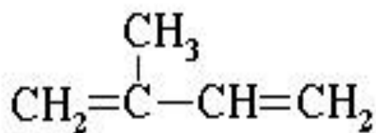
Изопрен
