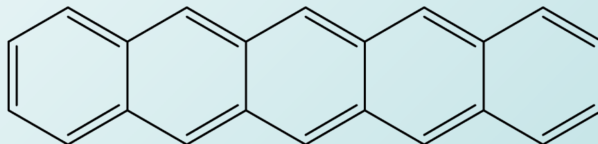
Пентацен
