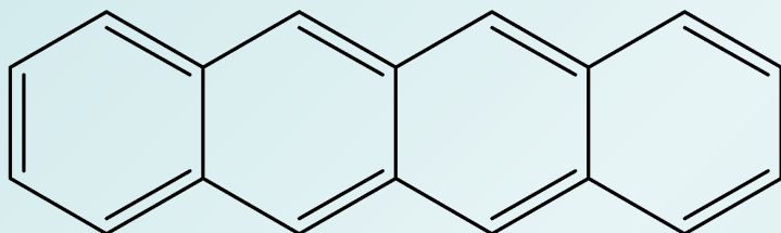
Тетрацен
