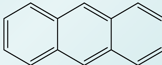
Антрацен
