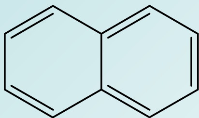
Нафталин
