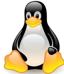
Linux
