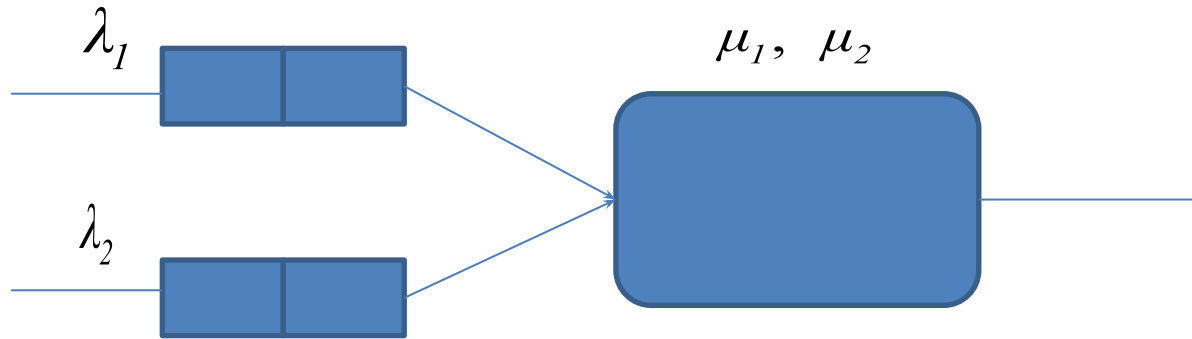
Рис. Одноканальная СМО
