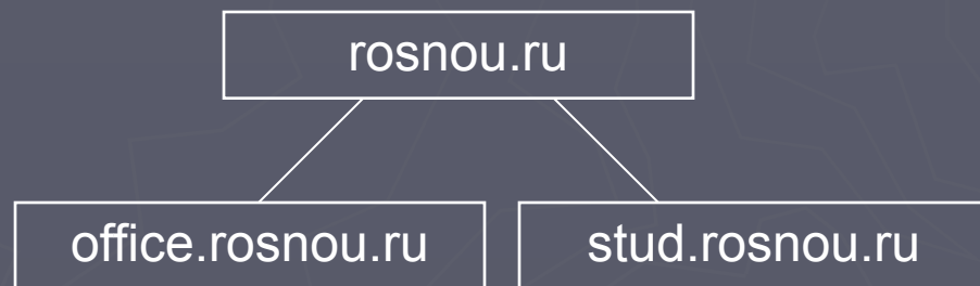
Дерево доменов
