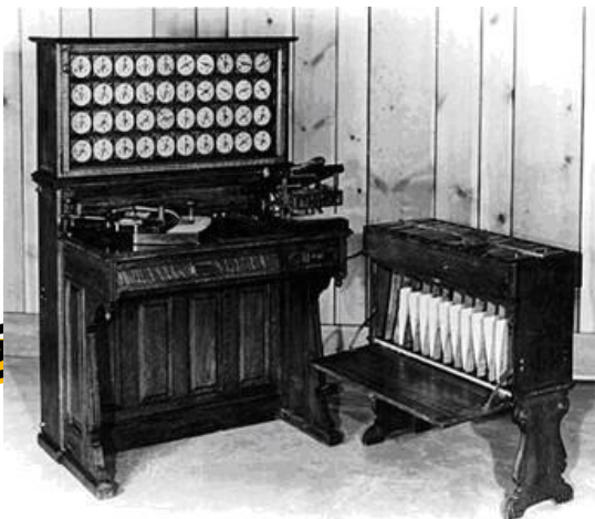
Табулирующая машина Г.Холлерита
