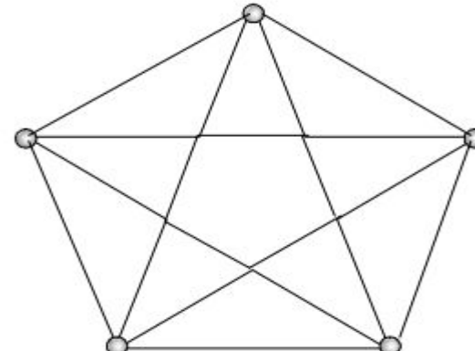
Рис. 3 – Сетевая БД
