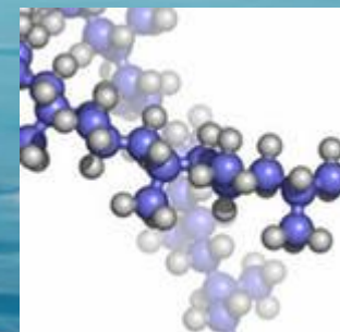
Молекула полипропилена
