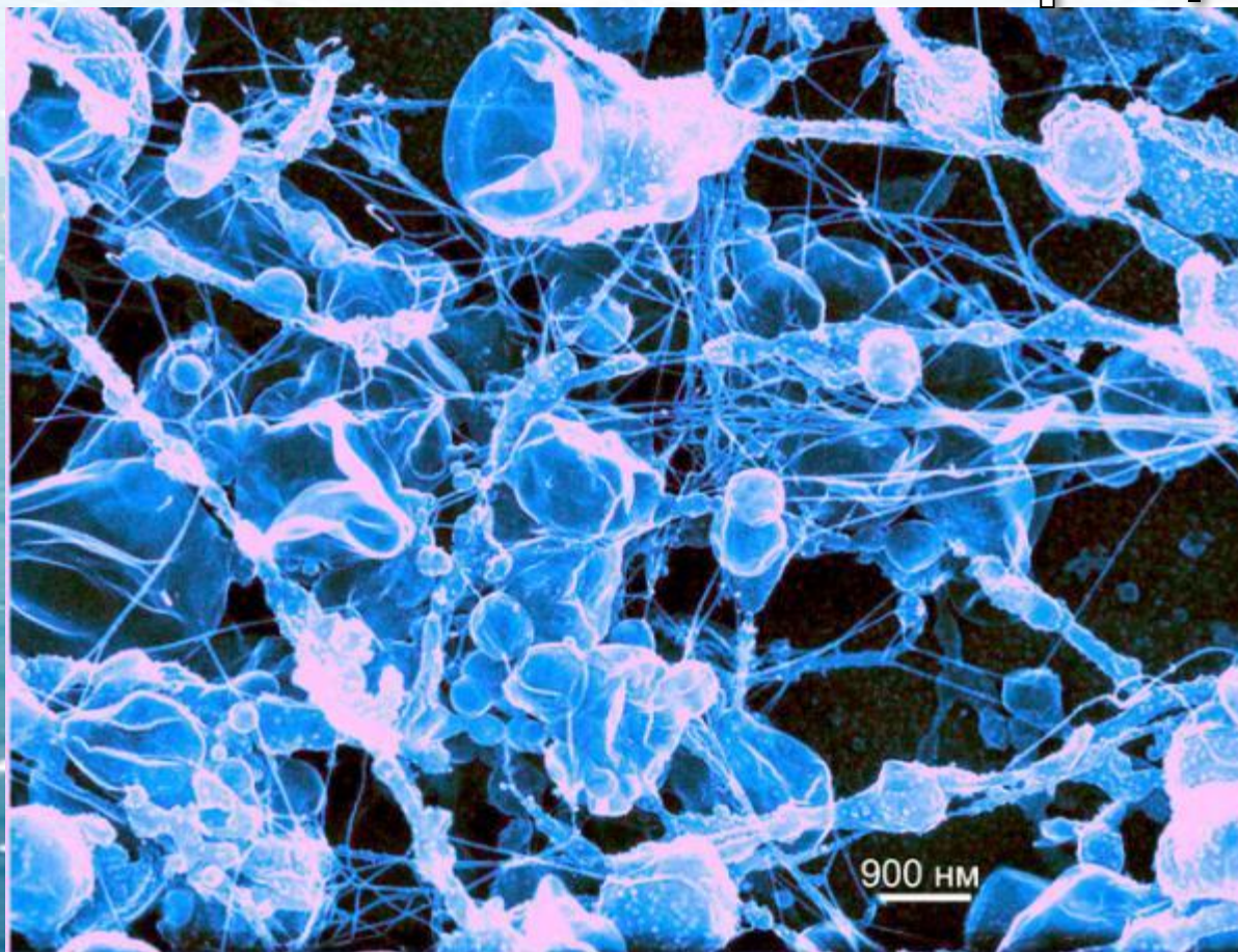
Молекула полипропилена
