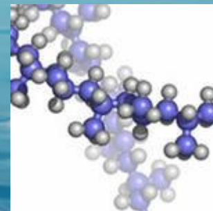
Молекула полипропилена
