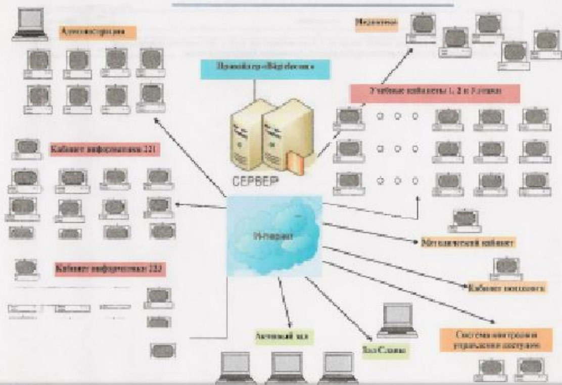
Схема локальной сети МБОУ СОШ №25 г.Химки
