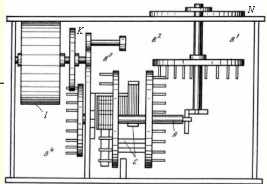
Элементы машины Паскаля, относящиеся к одному разряду числа
