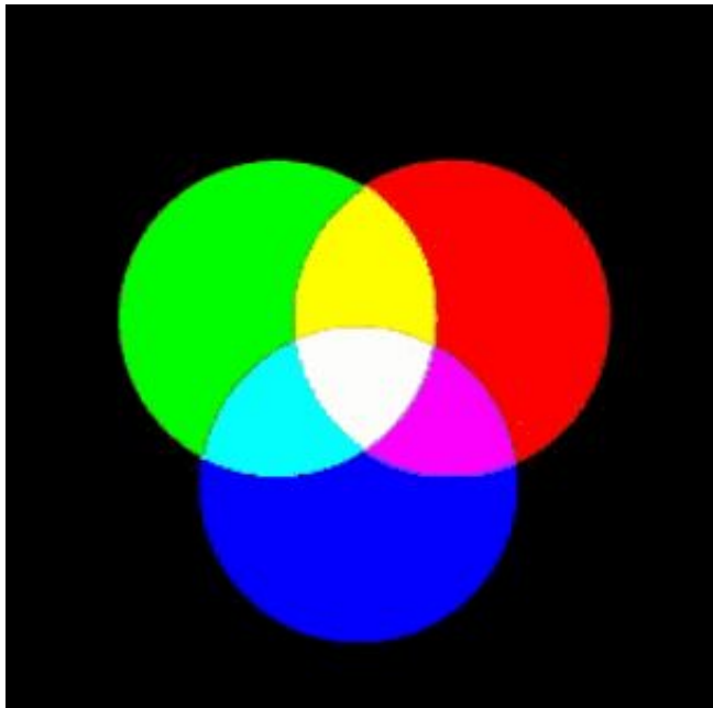
Схема цветообразования
