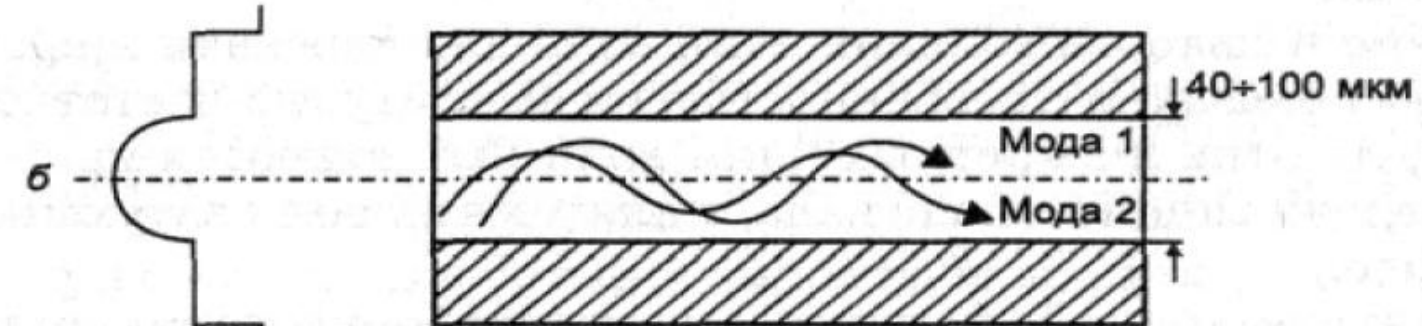
Многомодовое волокно с плавным изменением показателя преломления
