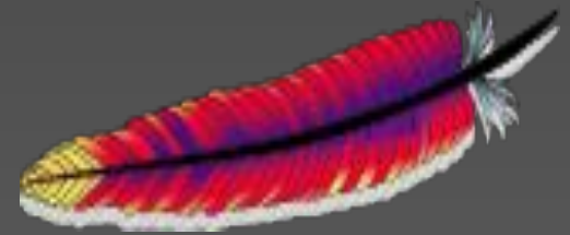
Логотип Apache
