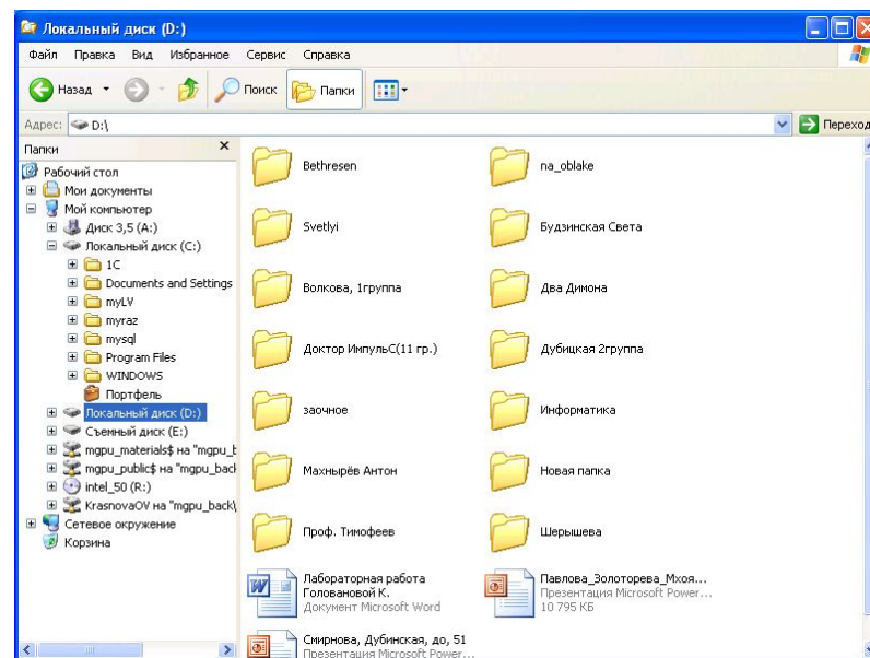
Окно Проводника
