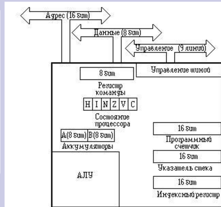
Рис 2.5 Микропроцессор MC6800 фирмы Motorola.
