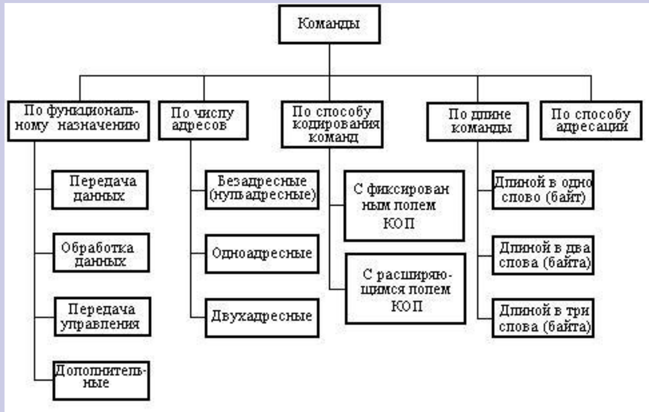
Рис. 2.3. Классификация команд.
