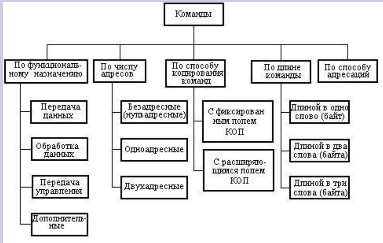
Рис. 2.3. Классификация команд.
