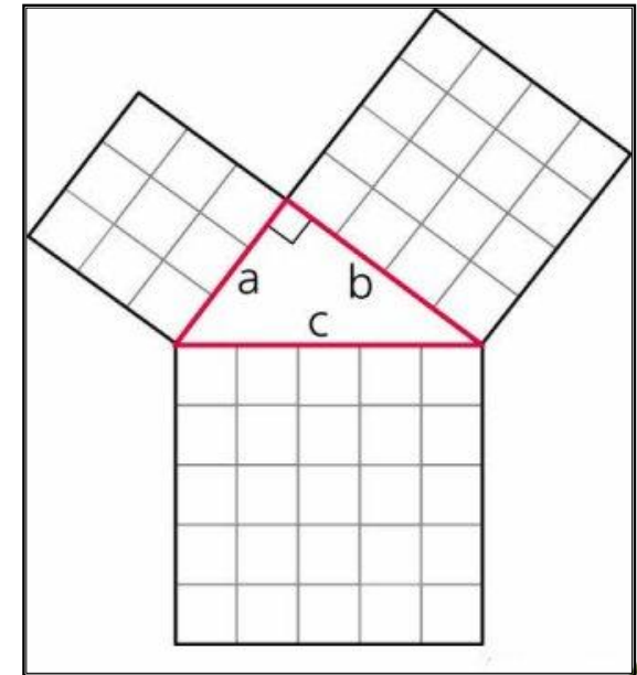
Теорема Пифагора
