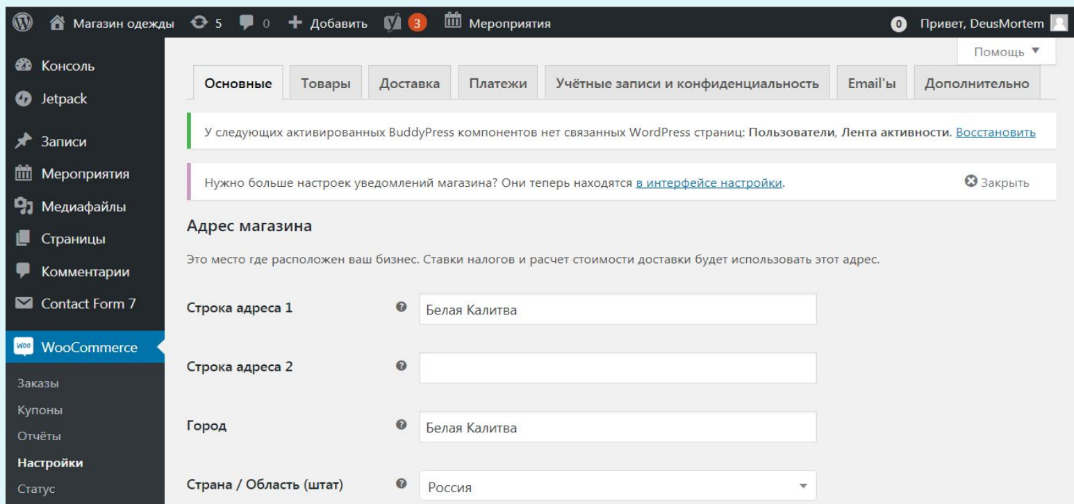
Рисунок 2.- Настройка WooCommerce
