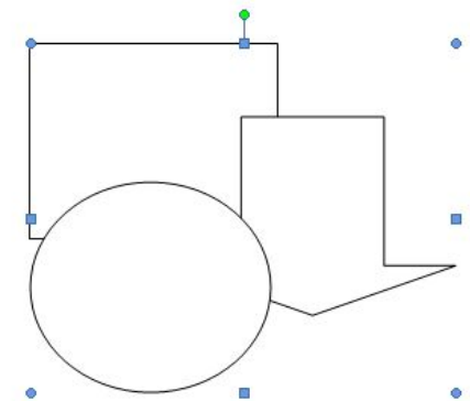
Сгруппированные фигуры
