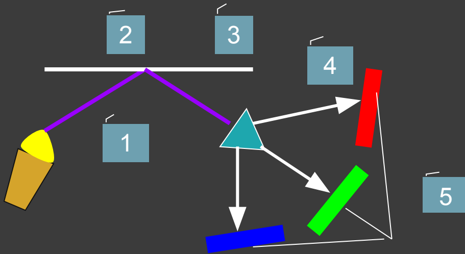
Рис. 5 Однопроходной сканер с призмой:
