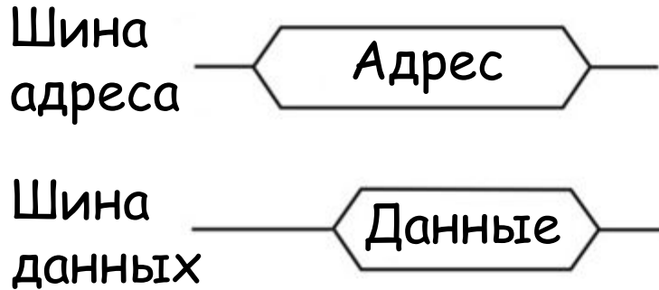
Немультиплексированные шины
