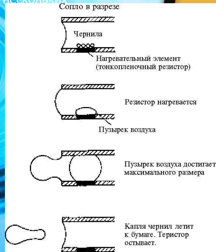
Принцип работы струйного принтера
