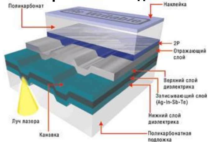
Строение DVD-диска
