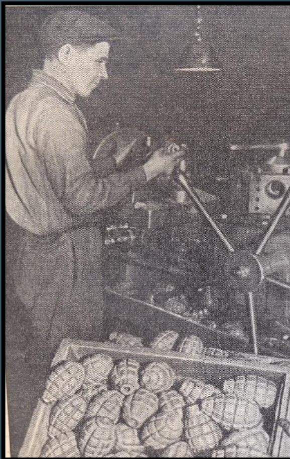
Обработка корпусов ручных гранат Ф-1 на одном из оборонных заводов
