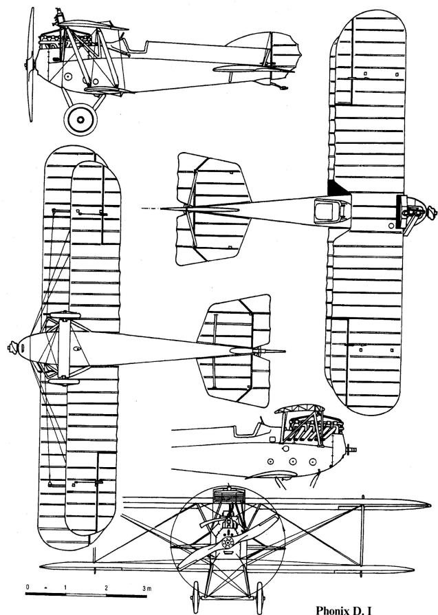
Phonix D. I
