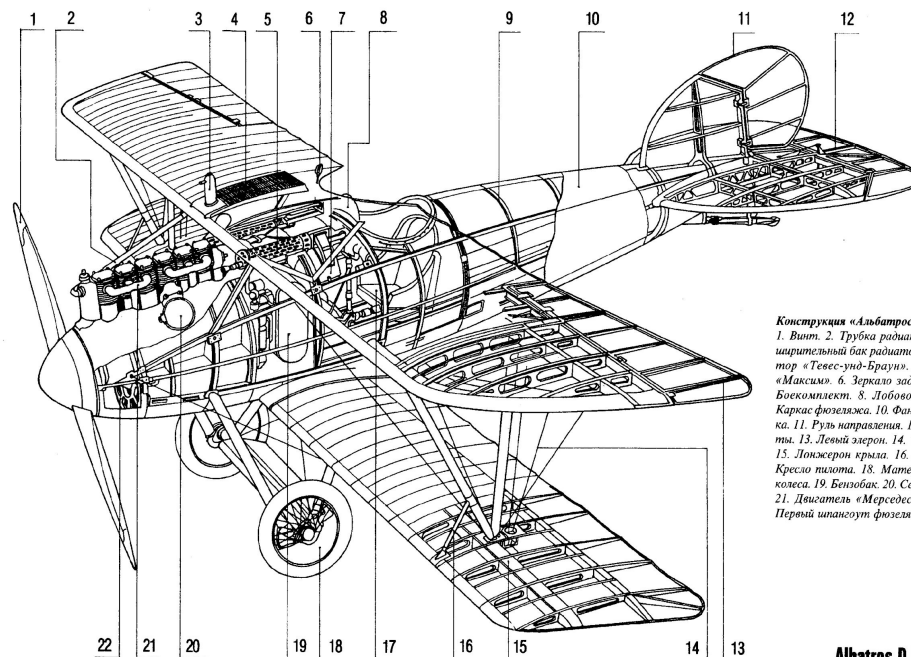
Albatros D.V
