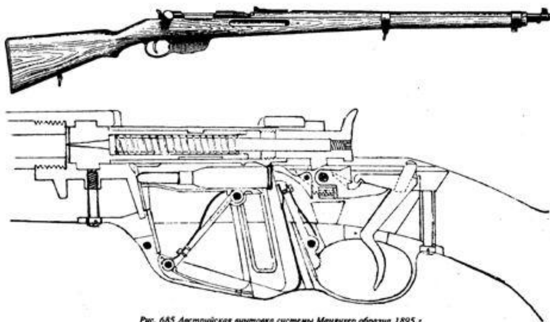
Рис. 685 Австрийская винтовка системы Манлихер образца 1895 г.
