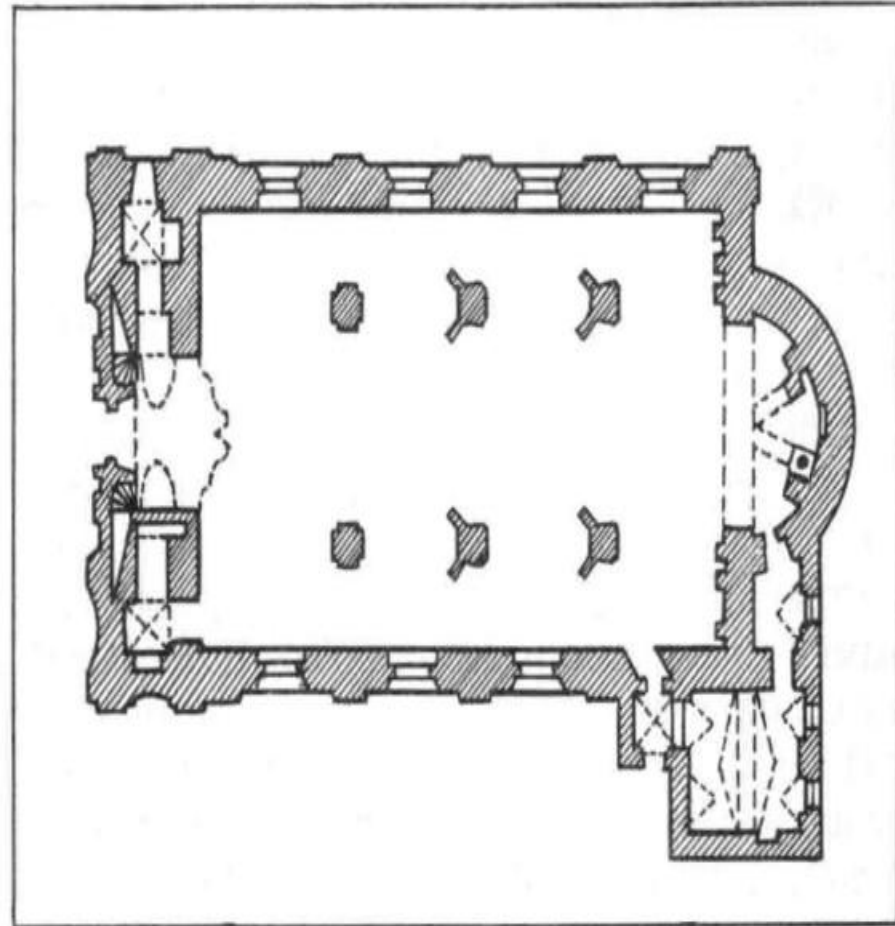
в. Васілішкі. Касцёл Іаана Хрысціцеля ордэна дамініканцаў. План.
