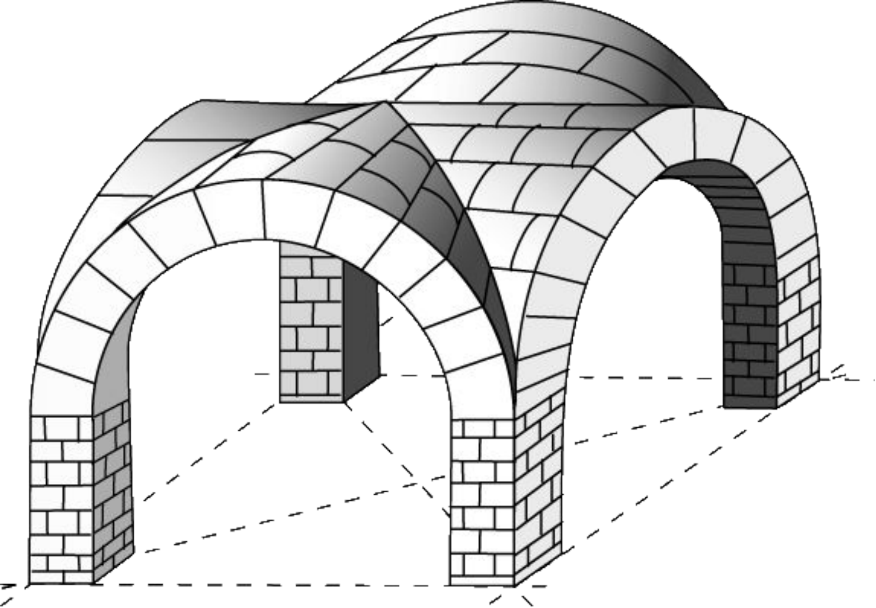
Схема крестового свода
