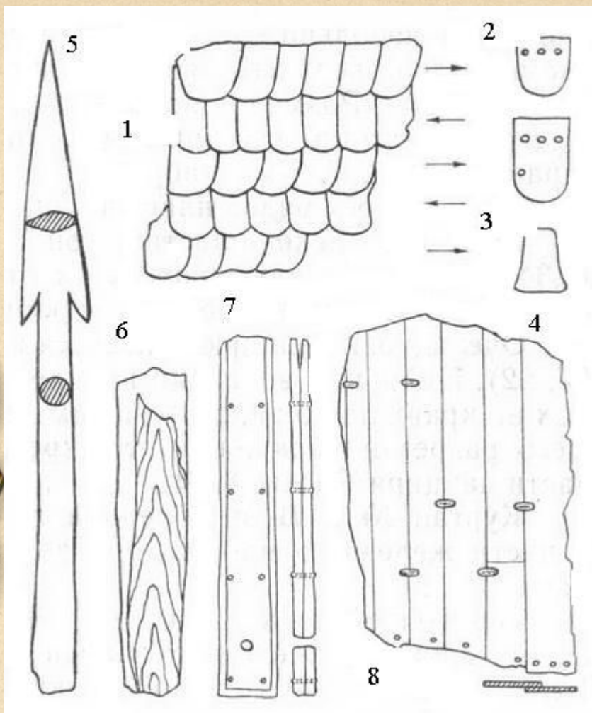
Панцирные пластинки (1-3) и ворварка (4) из Семибратних курганов. Кубань, Россия
