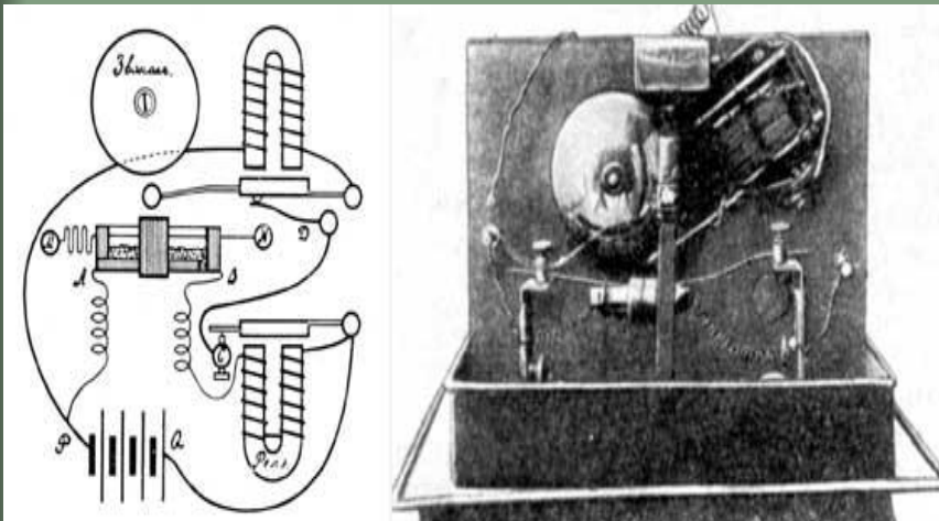
Приемник Попова
