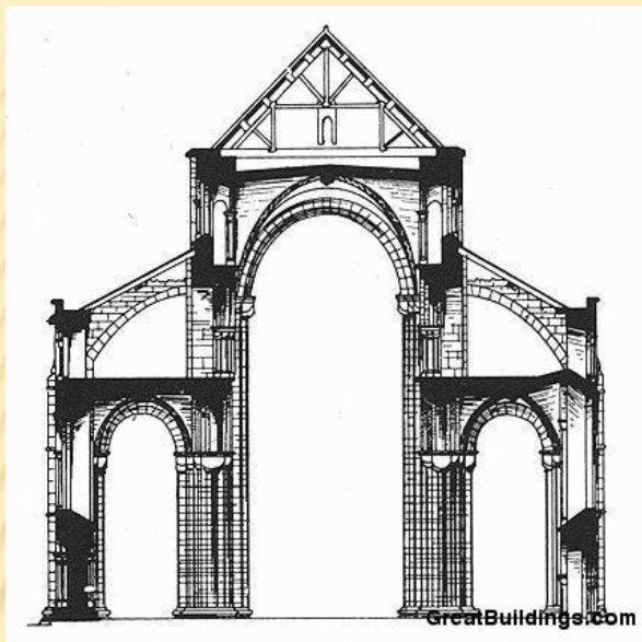
Романский храм в разрезе
