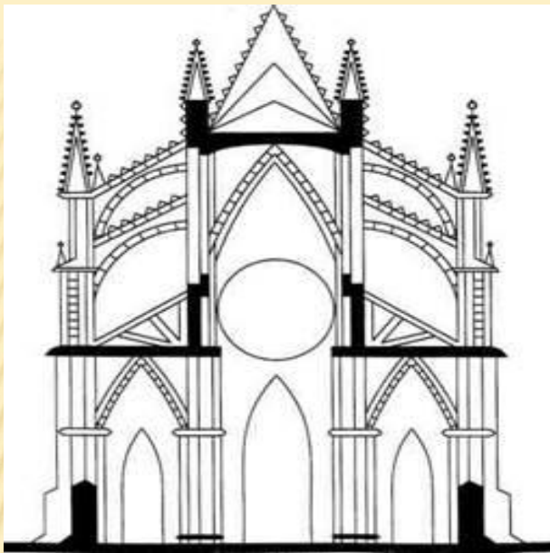
Готический храм в разрезе
