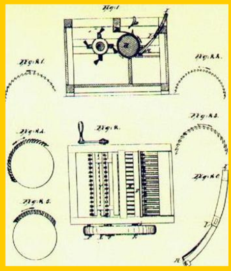
Э.Уитни и чертеж его машины
