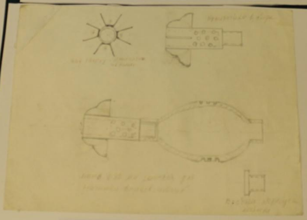
Чертеж срочного заказа особого назначения для фронта - стабилизатора для мины
