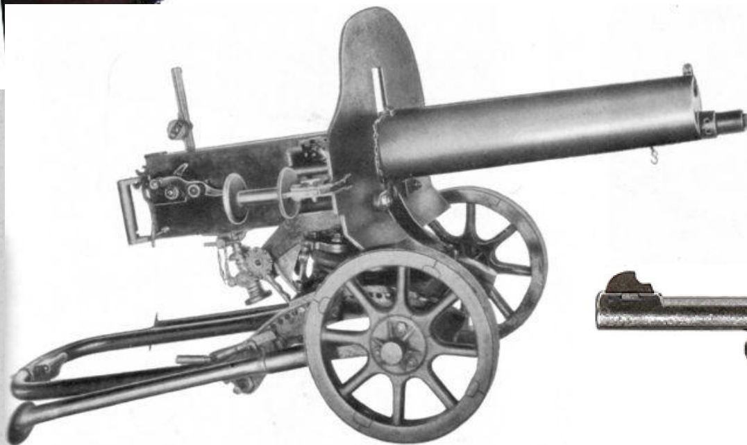
Станковый пулемёт системы Максима
