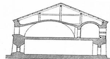
Разрез палаты
